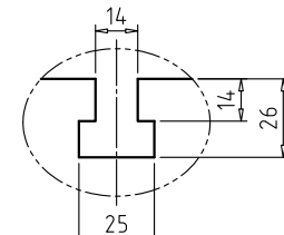
T-SLOT
