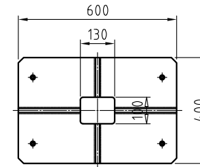
하판 볼스터
