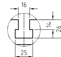
T-Slot
