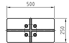
상판 볼스터
